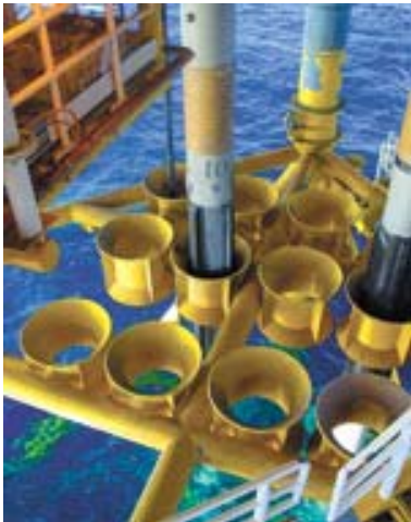
Centralisers
